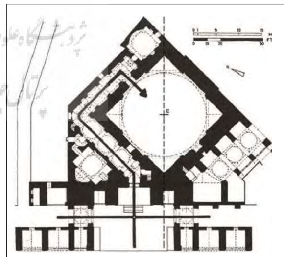
شکل ۲. پلان مسجد شیخ لطف الله (ماخذ: پیرنیا، ۱۳۸۳)
