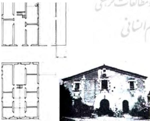
شکل ۱. پلان و نمای یک نمونه از گونه ماسیا (خانه کاتالانا) (Source: Le Corbusier, 1986)
