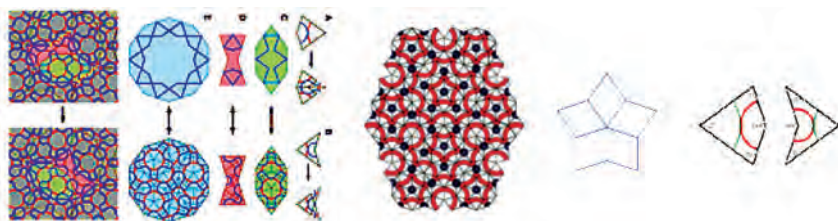
شکل ۲. از راست به چپ: اشکال کایت و دارت، تشکیل ستاره با کایت و دارت، چیدمان پنرز، تحلیل لو و هارت از شبه کریستالی بودن کاشیکاری کایت و دارت پنرز
