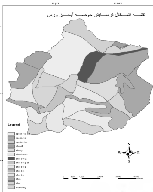
نقشه شماره ۸: نقشه اشکال فرسایش حوزه آبخیز ورس
