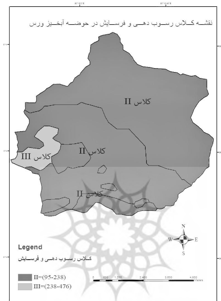
نقشه شماره ۱۱: کلاس‌های رسوب و فرسایش در حوضه ورس
