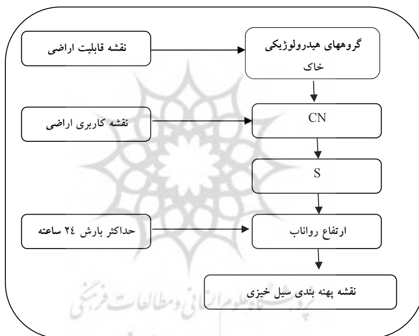
شکل ۳: نمودار جریان روش SCS استان گلستان
