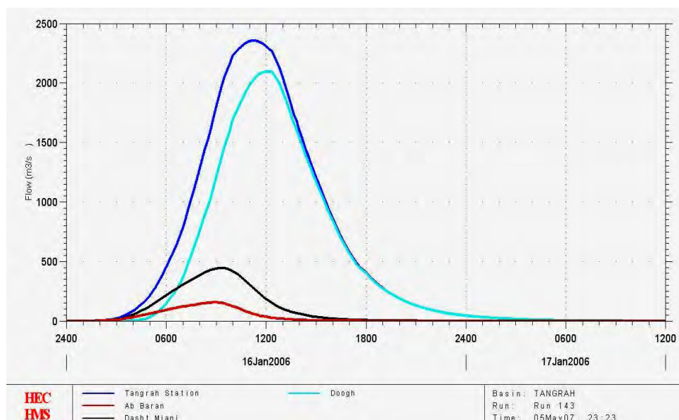
شکل ۲: هیدروگراف سیلاب برآورد شده برای ایستگاه تنگراه با دوره برگشت ۵۰ سال به روش SCS
