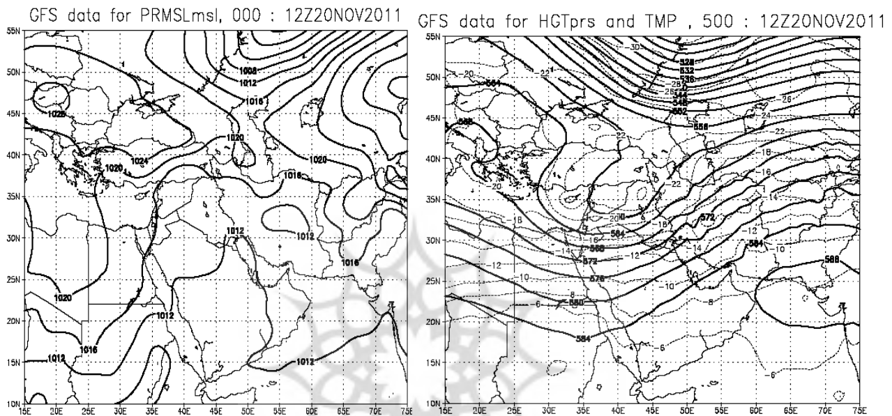
شکل ۵: الگوی فشارسطح زمین ساعت ۱۲ روز ۲۰ نوامبر
