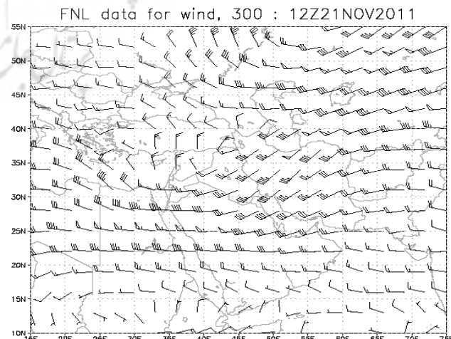
شکل ۱۲: آرایش سرعت و جهت باد در سطح ۳۰۰
