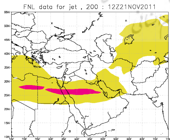
شکل ۱۱: نمایش هسته سرعت رودباد جنب حاره ای تراز ۲۰۰
