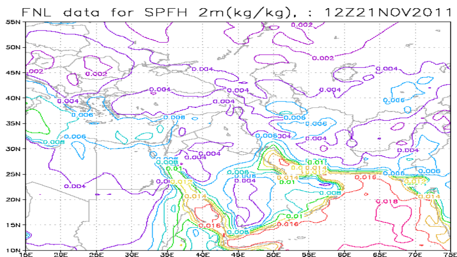
شکل ۱۰: الگوی نم ویژه ساعت ۱۲:۰۰ روز ۲۱ نوامبر
