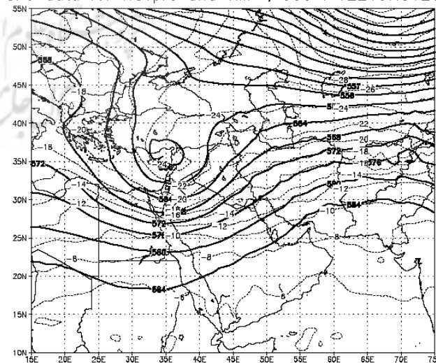
شکل ۳: نقشه تراز ۵۰۰ هکتوپاسکالی روز ۱۹ نوامبر ساعت ۱۲:۰۰
