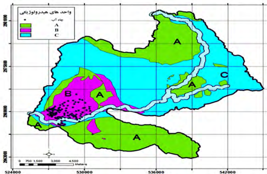
شکل ۱۰: واحد های هیدروژئومورفولوژی حوضه آبریز دشت گرو
