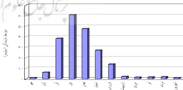
شکل ۴: تغییرات متوسط بارندگی ماهانه
