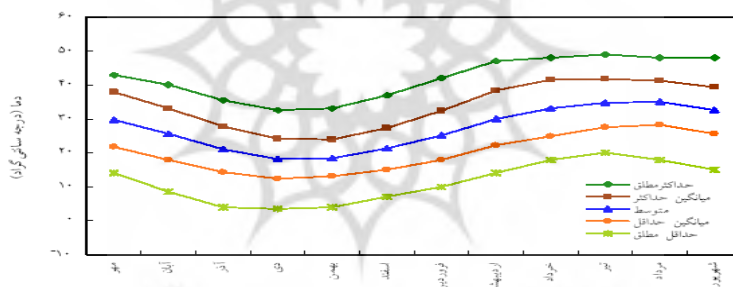
شکل ۳: تغییرات ماهانه شاخص های دما در ایستگاه مازابی
