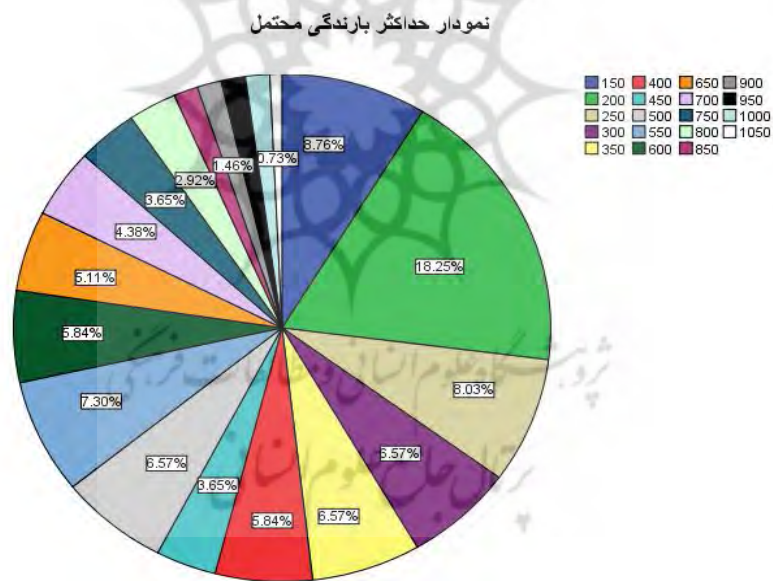
شکل ۶: نمودار مربوط به درصد فراوانی حداکثر بارندگی محتمل در ایران
