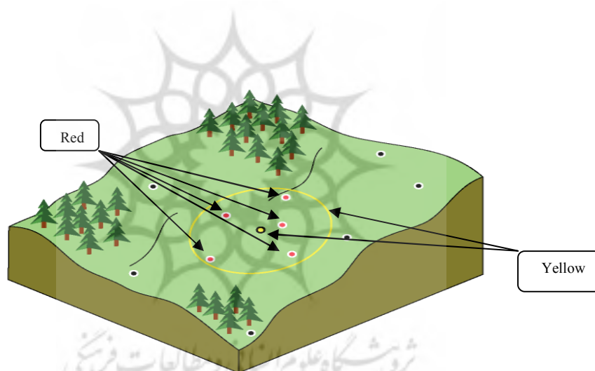
شکل ۳: وزن دهی بر اساس Kriging
