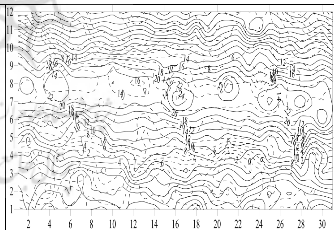
شکل ۹: میانگین حداقل دمای پیش بینی شده برای دوره ۲۰۰۷-۲۰۴۰
