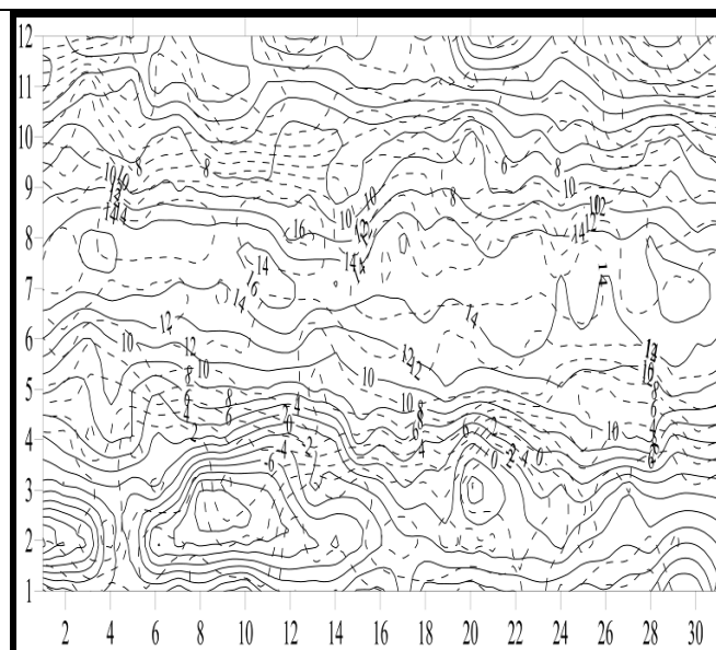
شکل ۴: میانگین دمای دوره سوم ۱۹۹۷-۲۰۰۱
