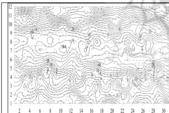
شکل ۷: میانگین حداکثر دمای پیش بینی شده برای دوره ۲۰۷۰-۲۰۴۱
