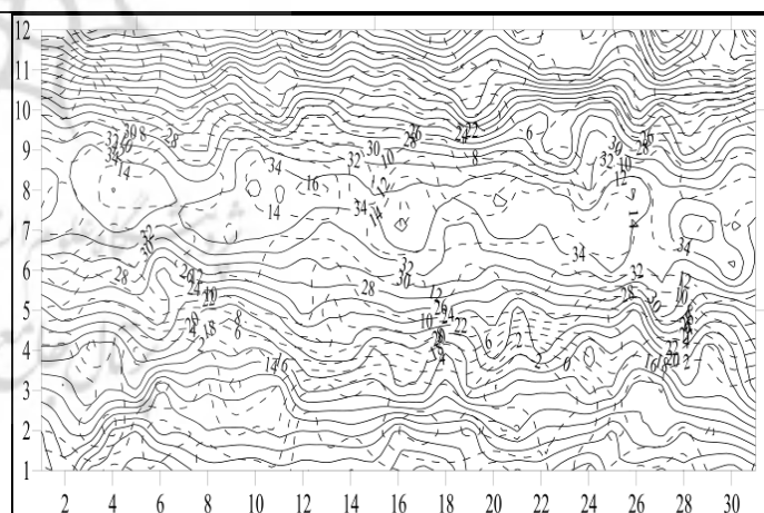
شکل ۶: میانگین حداکثر دمای پیش بینی شده برای دوره ۲۰۴۰-۲۰۱۱
