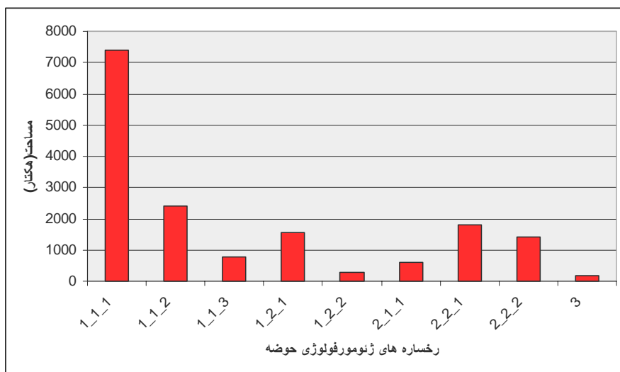
شکل (۳) نمودار ستونی مساحت رخصاره های ژئومورفولوژی
