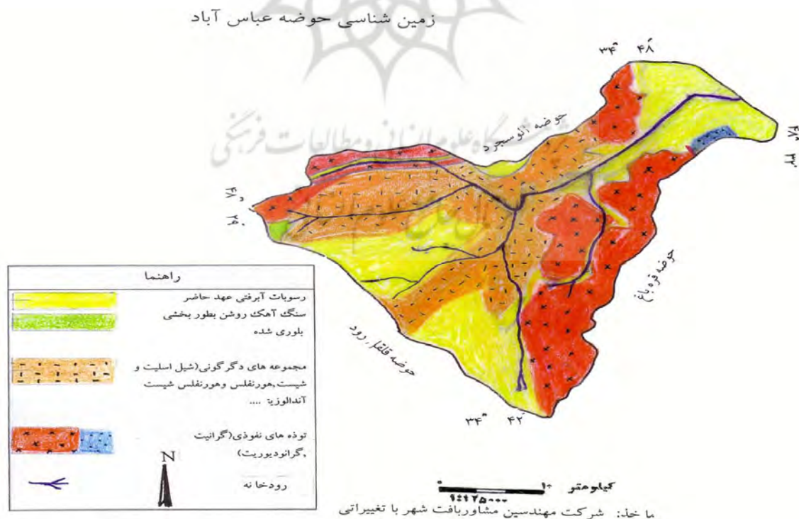
نقشه ۲ - زمین شناسی حوضه عباس آباد
