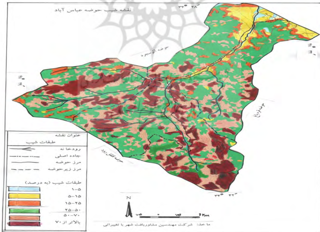
نقشه ۳ - طبقه‌بندی شیب حوضه عباس آباد
