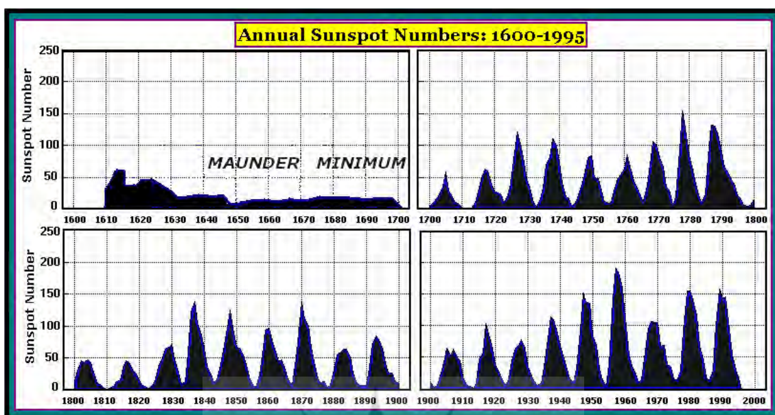
شکل ۵- تعداد سالانه و سیکل لکه‌های خورشیدی از ابتدای قرن هفدهم (Barry&Chorley,2003)
