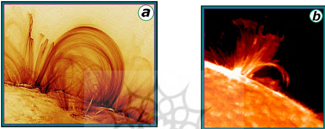
شکل ۱- شکل‌های ۱a و ۱b به ترتیب خطوط میدان مغناطیسی بسته و شراره خورشیدی را در یک منطقه‌ی فعال از خورشید نشان می‌دهند. (منبع: http://www.gsfc.nasa.gov/gsfsc/spacesci/pictures/ )
