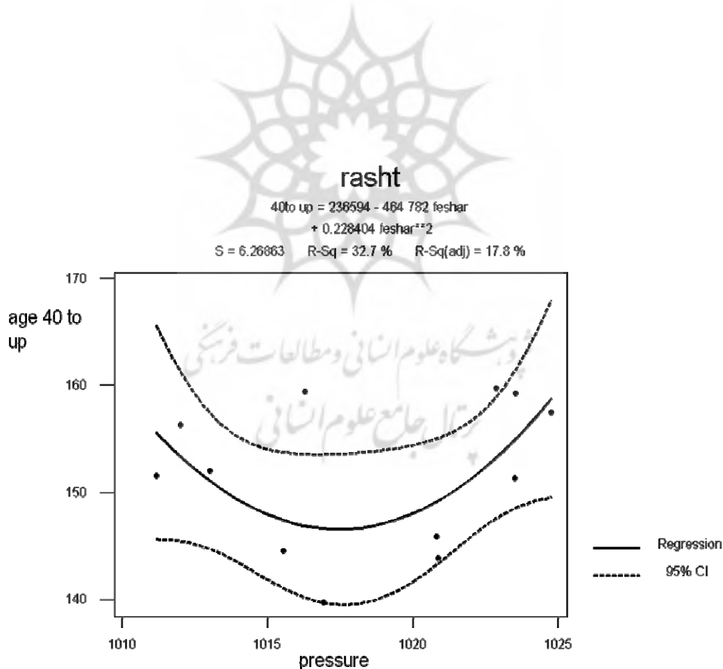
شکل ۱- شناسایی میزان مطلوبیت فشار هوا در رشت با بیماری قلبی از همبستگی رگرسیون غیر خطی
