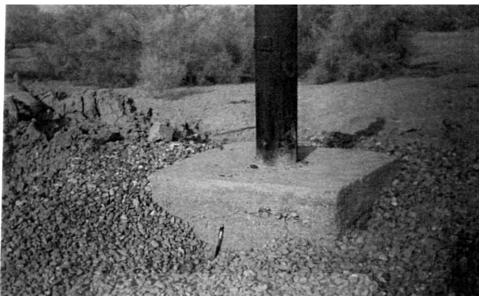
شکل ۴ - بالا زدگی فونداسیون لوله چاه ایستگاه تثبیت ماسه شهید صدوقی
