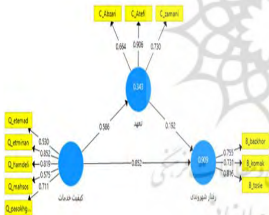
نمودار ۱: برازش مدل اندازه گیری تحقیق
