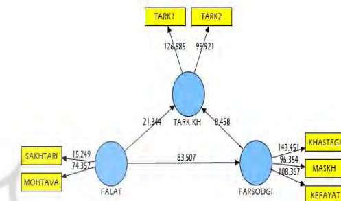
شکل ۲. خروجی نرم افزار پی ال اس در حالت معنی داری
