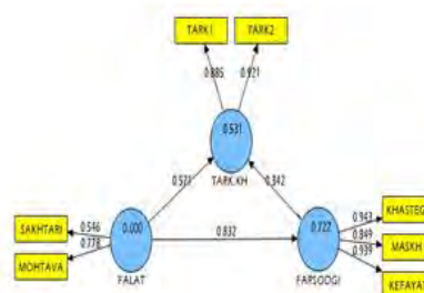
شکل ۱. خروجی نرم افزار بی ال اس در حالت استاندارد
