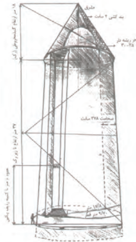
شکل ۵. مشخصات و اندازه هندسی برج قاپوس، (مأخذ: معطوفی، ۱۳۹۰)
