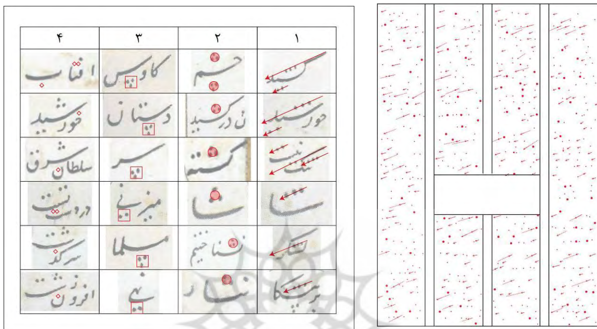
تصویر ۱۷- پراکندگی انرژی نقطه‌ها در یک صفحه، مأخذ: نگارندگان
