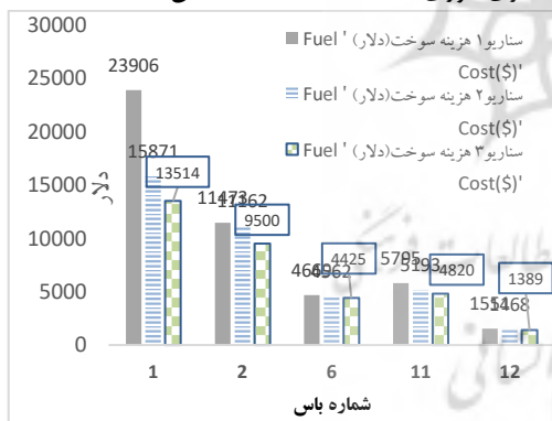
نمودار ۱۹. مقایسه سه سناریو از نظر مقدار هزینه سوخت در ۲۴ ساعت
