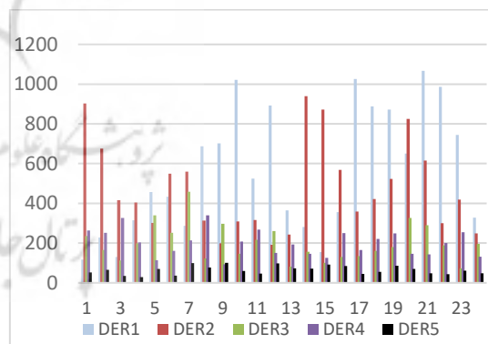
نمودار ۱۷. سوخت مصرفی دیزل‌ها در سیستم ۱۴ باسه طی ۲۴ ساعت شبانه‌روز تحت سناریوی ۳
