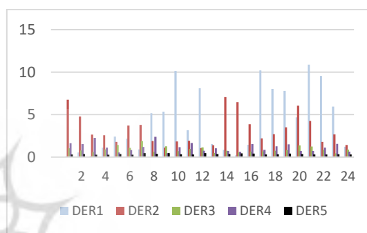
نمودار ۱۶. آلاینده‌گی تولیدی دیزل‌ها در ریز شبکه در طی ۲۴ ساعت شبانه‌روز تحت سناریوی ۳
