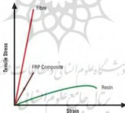
شکل ۳ منحنی تنش-کرنش الیاف شیشه، رزین FRP
