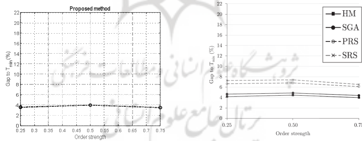
شکل 1. خروجی روش پیشنهادی فاصله T_{min} برای مقادیر متفاوت توان ترتیبی (OS) و پژوهش [9]
