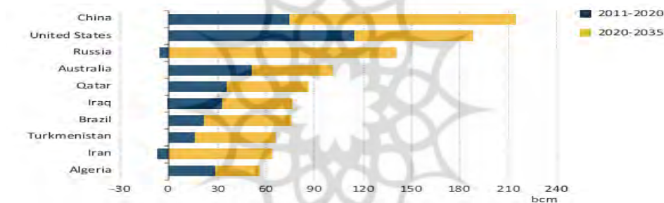
نمودار (۱). تغییر در تولید گاز طبیعی سالانه در کشورهای منتخب در سناریو جدید
