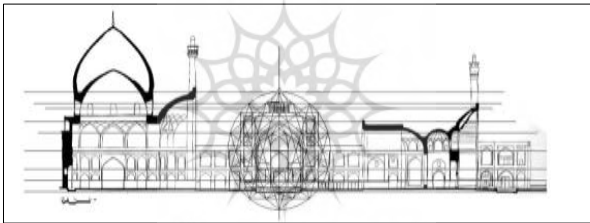
تصویر ۶. تحلیل هندسی ایوان شرقی مسجد امام اصفهان بر مبنای تناسبات طالپی ( پنج ضلعی منظم منبع: مهدی زاده سراج، ۱۳۹۳: ۱۵)
