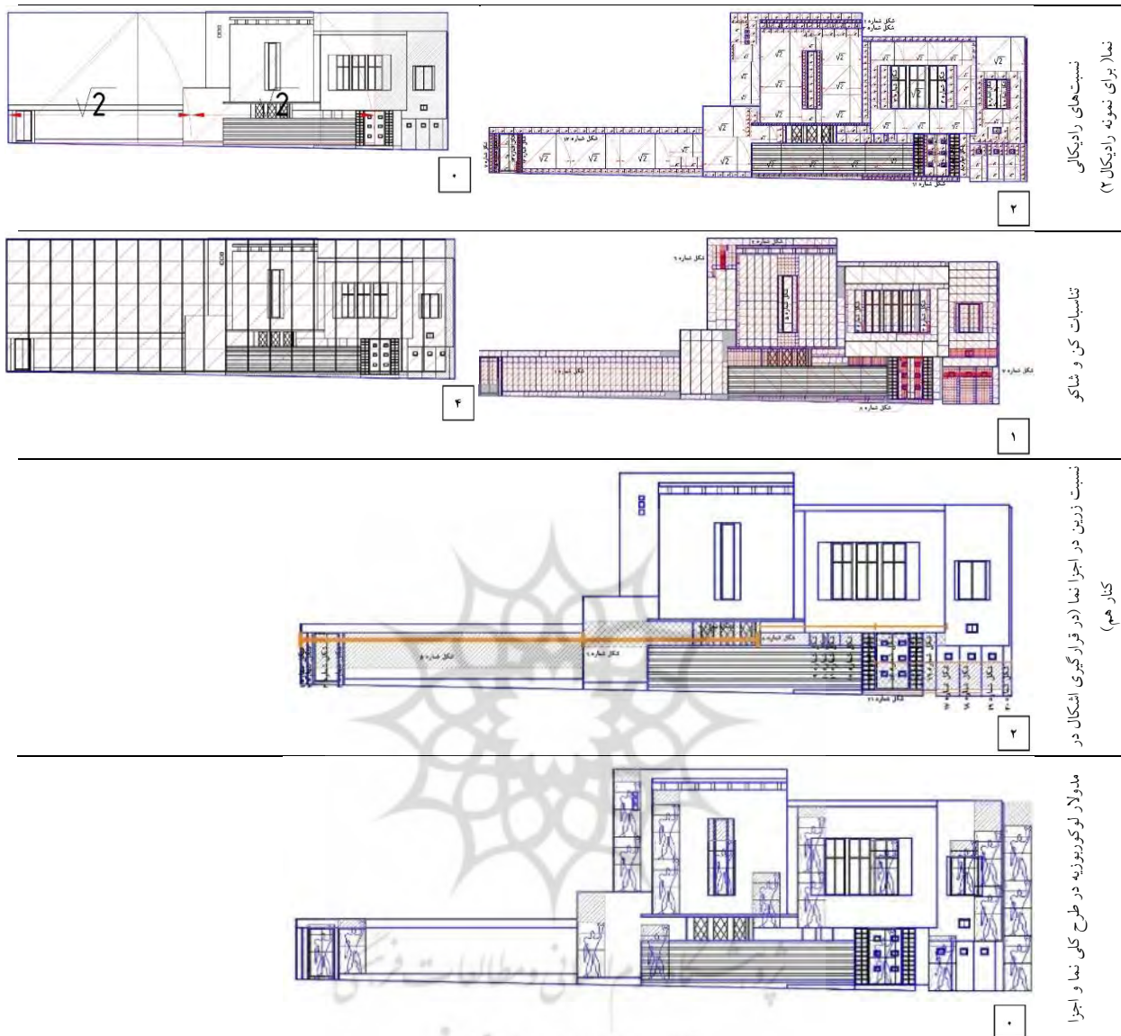
تصویر ۱۲: تحلیل‌های تناسباتی نمای اصلی خانه میردامادی (منبع: یافته‌های پژوهش، ۱۳۹۹)
