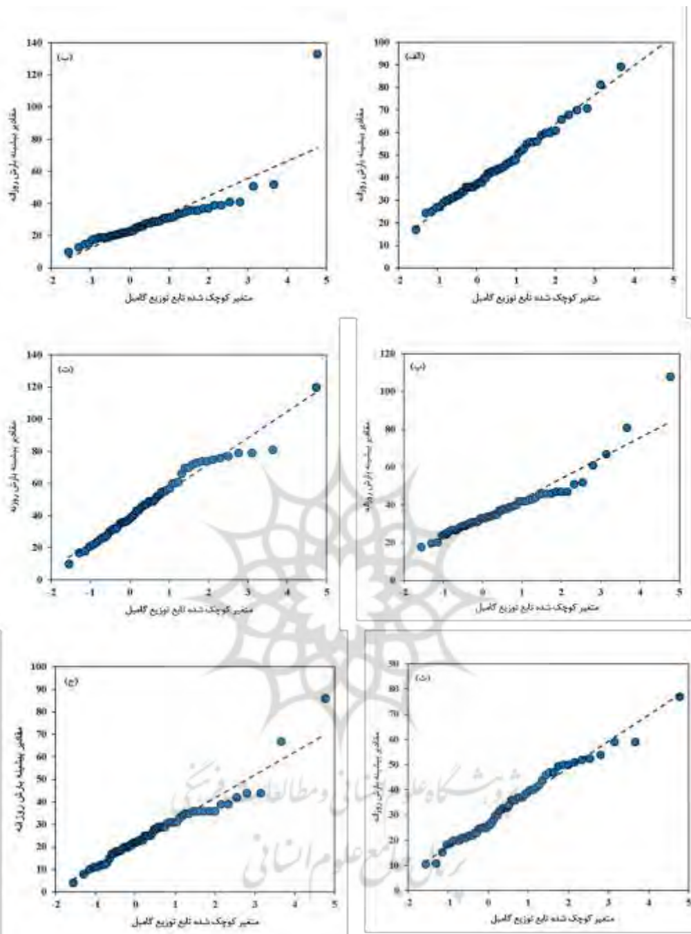
شکل ۳. نمودار پراکندگی بیشینه سالانه بارش در مقابل متغیر کوچک شده توزیع گامبل: الف) ایستگاه سینوپتیک خرم‌آباد، ب) همدان، پ) کرمانشاه، ت) دزفول، ث) اهواز، ج) آبادان
