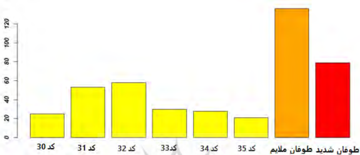
شکل ۲. تعداد طوفان‌های گرد و غبار در ایستگاه سبزوار
