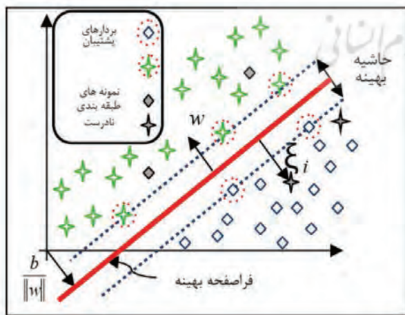
نگاره ۳: فاصله بهینه جداکننده دو کلاس در الگوریتم ماشین‌های بردار پشتیبان (صمدزادگان و فردوسی، ۱۳۹۲)
