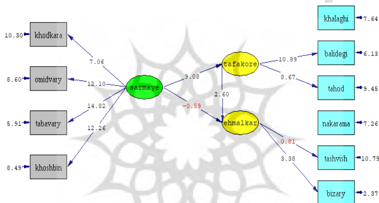
شکل ۷. مدل اصلاح شده پژوهش در حالت ضرایب معنی داری (Value-t)
