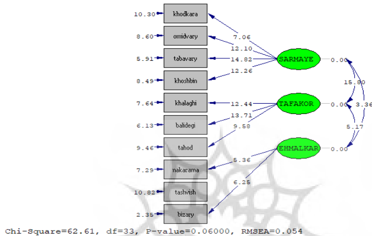
شکل ۳. بارهای عاملی آماره t تحلیل عاملی تائیدی
