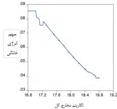
نمودار ۴- منحنی انگل ناپارامتریک برای سهم انرژی خانگی
