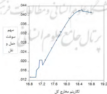
نمودار ۳- منحنی انگل ناپارمتریک برای سهم سوخت‌های حمل و نقل (منبع: یافته‌های پژوهشگر)
