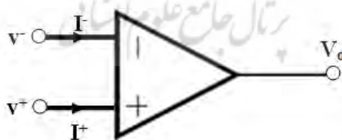
شکل ۳. آپ‌امپ ایده‌آل
