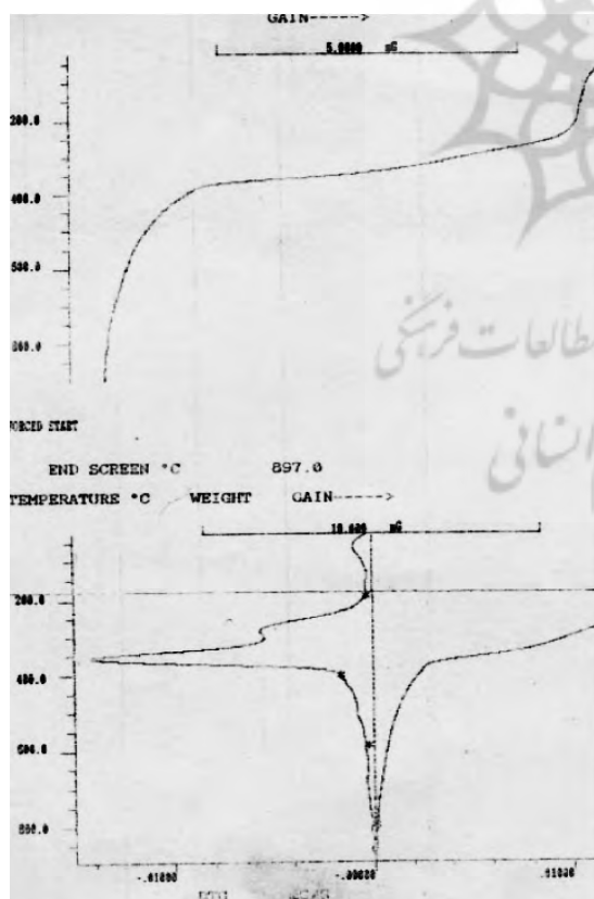
تصویر ۸. نمودار DTG نمونه درمان شده با محلول هیدروکسید باریم که نمونه یک پیرولیز در دمای 354^{\circ}\text{C} دارد (با یک اختلاف دمای 6/8^{\circ}\text{C} (+) نسبت به نمونه شاهد)
