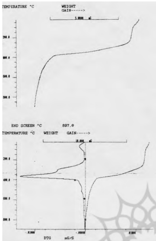
تصویر ۱۰. نمودار DTG نمونه درمان شده با نانو ذرات هیدروکسید منیزیم. پیک پیرولیز سلولز در ۳۶۷/۳ رخ می‌دهد (با یک اختلاف دمایی 22^{\circ}\text{C} + نسبت به نمونه شاهد).
