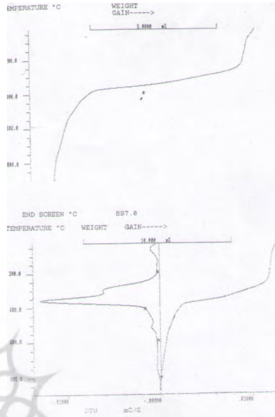
تصویر ۹. نمودار DTG نمونه درمان شده با نانو ذرات هیدروکسید کلسیم. پیک پیرولیز سلولز در دمایی ۳۵۸/۷ رخ می‌دهد (با یک اختلاف دمایی 13^{\circ}\text{C} + نسبت به نمونه شاهد).
