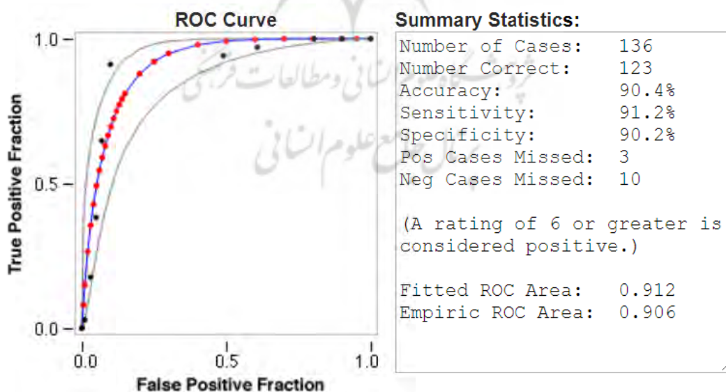
شکل ۳. منحنی ROC
