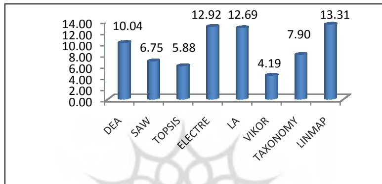
نمودار ۹. همبستگی بین رتبه حاصل از روش‌های ادغامی
