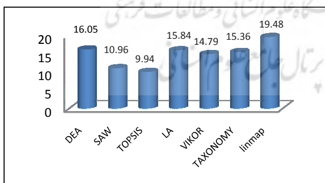
نمودار ۳. اختلاف رتبه روش ELECTRE با سایر روش‌ها
