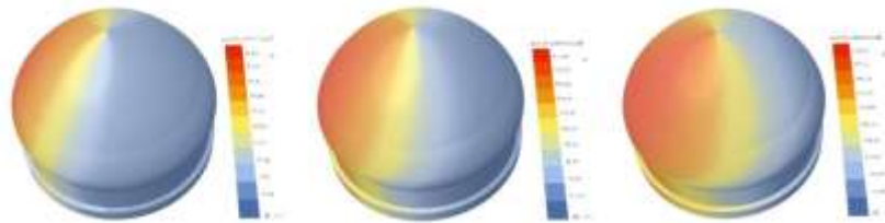
تصویر ۱۰: دریافت تابش خورشید بر سطوح گنبد مساجد تک پوسته، در بازه زمانی مختلف از راست به چپ ۱۴، ۱۶ و ۱۸ بعد از ظهر (وثیق و شیری، ۱۳۹۸)
