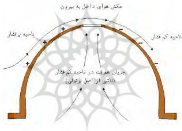
تصویر ۹: مکش هوا در گنبد طبق اصل برنولی (بهار، ۱۳۹۵)
