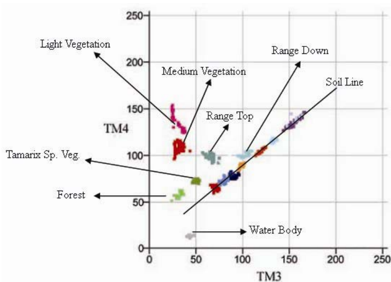
شکل ۴- نمایش پدیده های مختلف در فضای دویبعدی بین باندهای قرمز و مادون قرمز نزدیک
