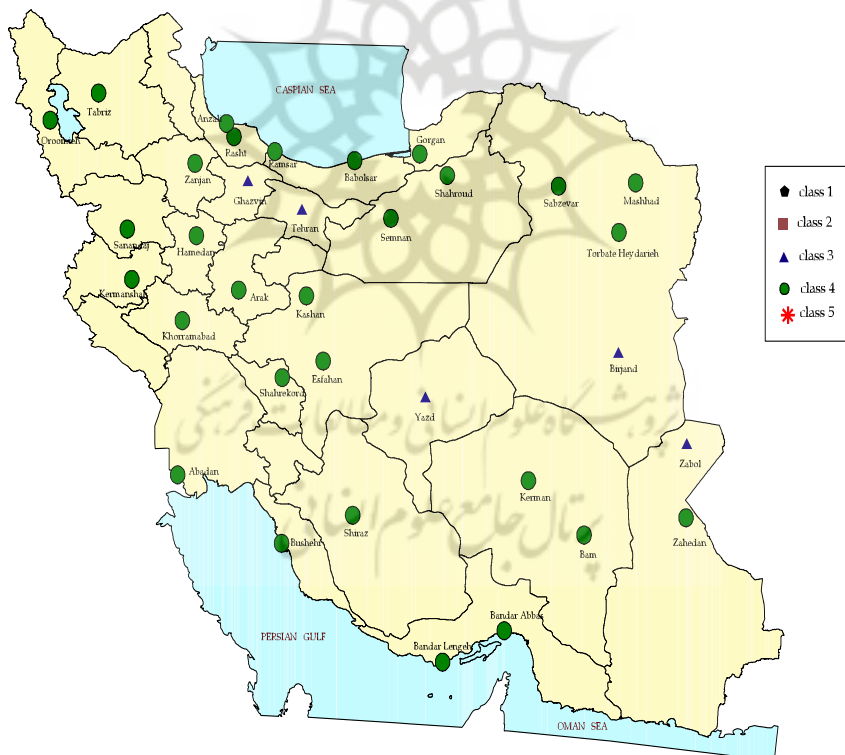
شکل ۱- کلاس همگنی سری های بارش ایستگاههای سینوپتیک کشور
