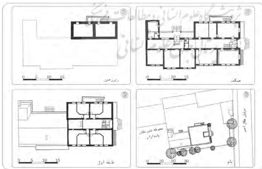
تصویر ۴: پلان‌های وضع موجود
