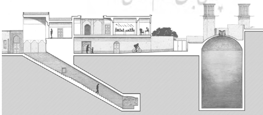
تصویر ۱۴: برش طولی از آب‌انبار وقت و ساعت یزد؛ ترسیم از سعید حسینی
