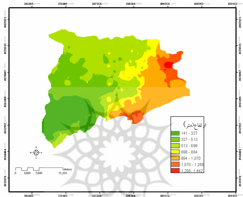
شکل ۵- درون یابی ارتفاع در حوضه سد گلستان ۲ بر اساس مدل IDW
