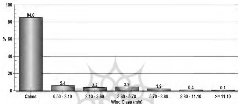
شکل (۴). توزیع تندی باد استان اصفهان در بازه زمانی بین ۲۰۰۴ تا ۲۰۱۶ (منبع: نگارندگان).
