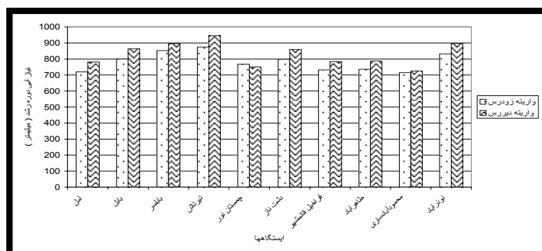
شکل ۷- نمودار نیاز خالص آبیاری دوره رشد وارپته های زودرس و دیررس برنج در ایستگاه های جلگه مازندران (۱۹۷۰-۱۹۹۹)
