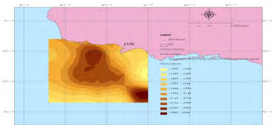
شکل ۸- مدل سازی مکانی میانگین سرعت جریان ناشی از باد (m/s) در ماه فروردین از فصل بهار
