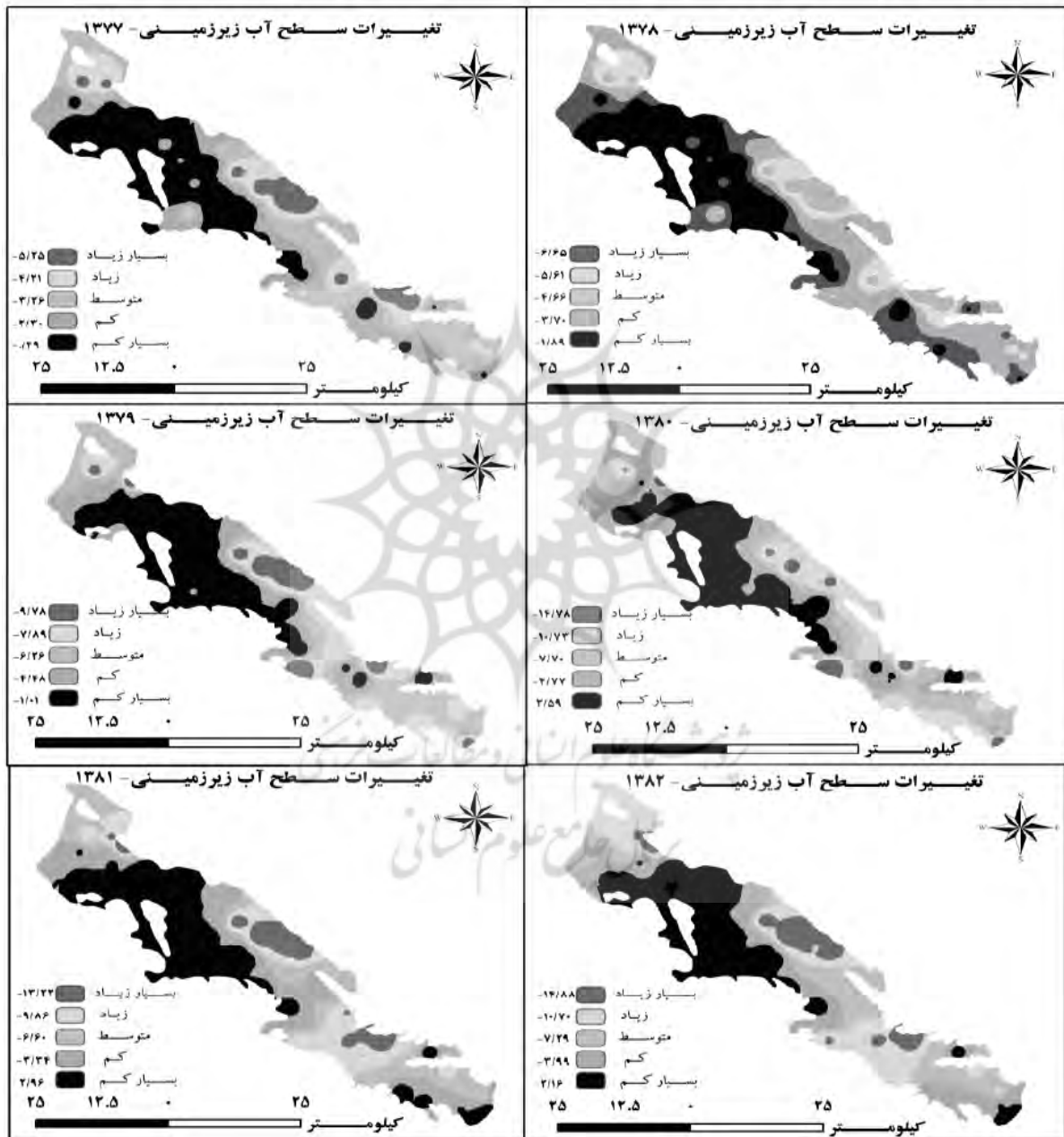
شکل شماره (۴): پهنه بندی میزان کاهش سطح آبهای زیرزمینی دشت نمدان (۱۳۸۲ - ۱۳۷۷) به متر
