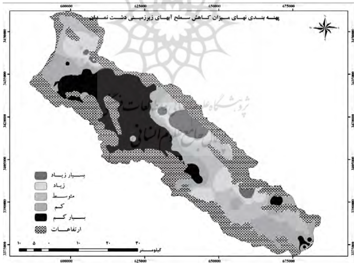
شکل شماره (۶): پهنه بندی نهایی میزان کاهش سطح آبهای زیرزمینی دشت نمدان
