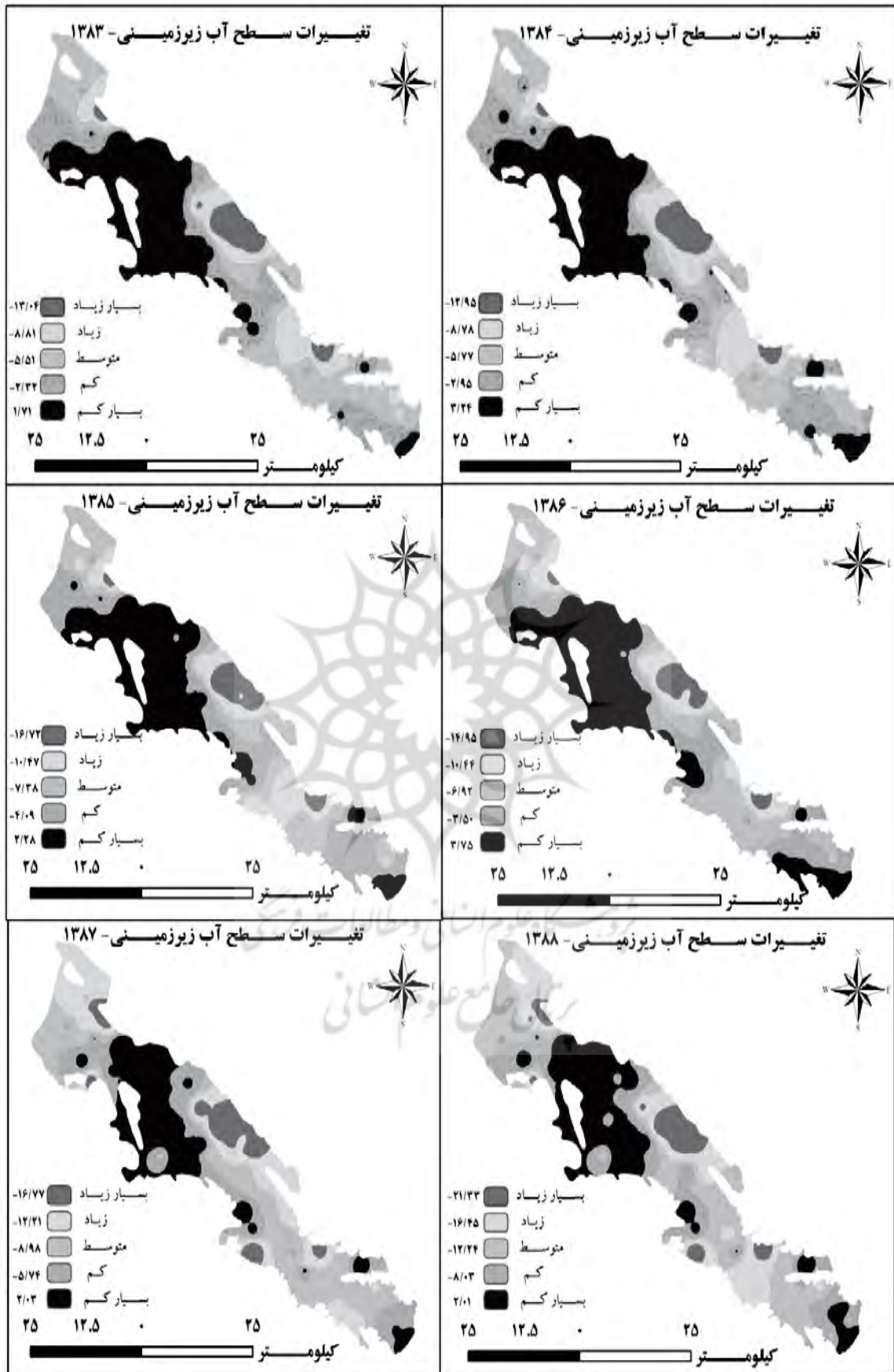
شکل شماره (۵): پهنه بندی میزان کاهش سطح آبهای زیرزمینی دشت نمدان (۱۳۸۳-۱۳۸۸) به متر
