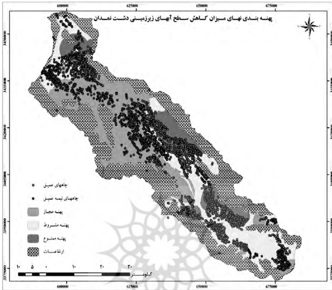
شکل شماره (۷): پهنه‌های نهایی تعیین شده جهت برداشت از آبهای زیرزمینی
