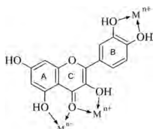
شکل ۸- ساختار اسکلتی فلاونوئیدها (راست) و مکان‌های احتمالی ترکیب یک فلز با ساختار مولکولی کوئرستین (چپ)
