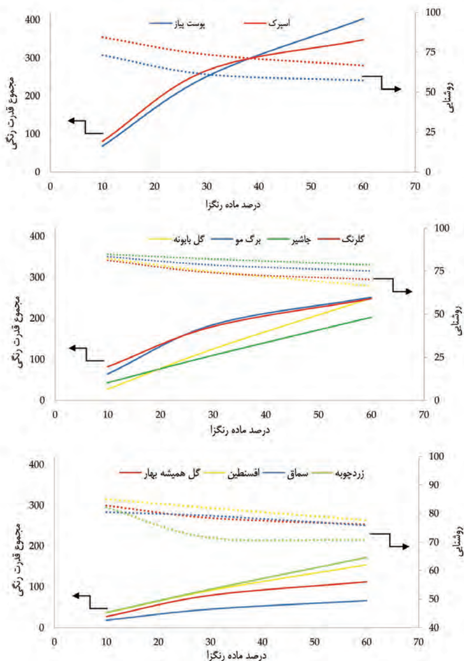
شکل ۷- نمودارهای مجموع قدرت رنگی نمونه کلاف‌های نخ پشمی رنگزای شده با درصدهای مختلف رنگزا در سه گروه با قدرت رنگی بالا، متوسط و کم
