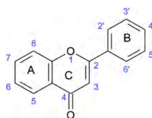
شکل ۸- ساختار اسکلتی فلاونوئیدها (راست) و مکان‌های احتمالی ترکیب یک فلز با ساختار مولکولی کوئرستین (چپ)
