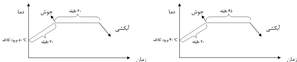
شکل ۳- نمودار فرایند دندان‌دانه دادن (سمت راست) و رنگ‌رزی (سمت چپ) به روش پیش دندان‌دانه
