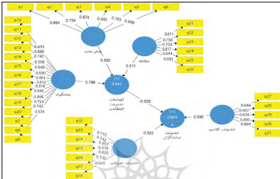
شکل ۱. تحلیل عاملی تأییدی مدل روابط بین متغیرهای تحقیق (ضریب مسیر)
