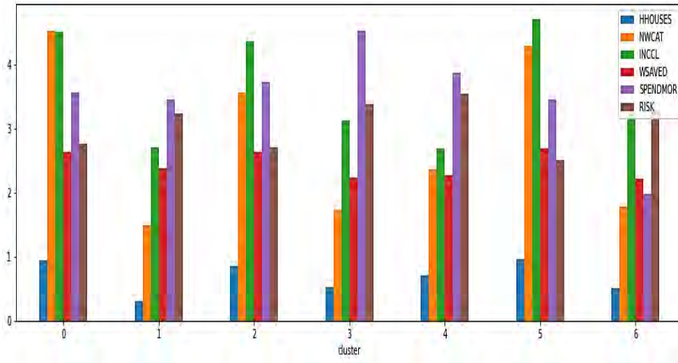
شکل ۷- خوشه‌بندی بر اساس ویژگی‌های مالی و ویژگی‌های مربوط به تمایل به ریسک. Figure 7- Clustering based on financial characteristics and risk-related characteristics.
