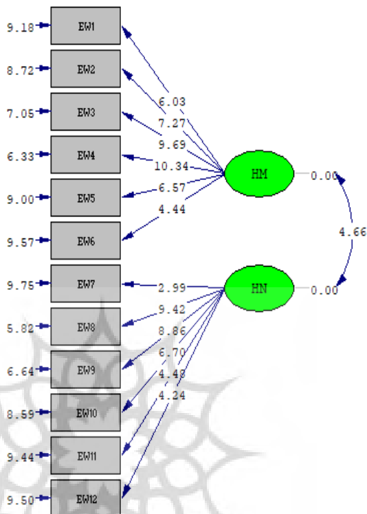
شکل ۳. آماره معناداری (t-value) تحلیل عاملی تأییدی پرسش‌نامه بهزیستی هیجانی
