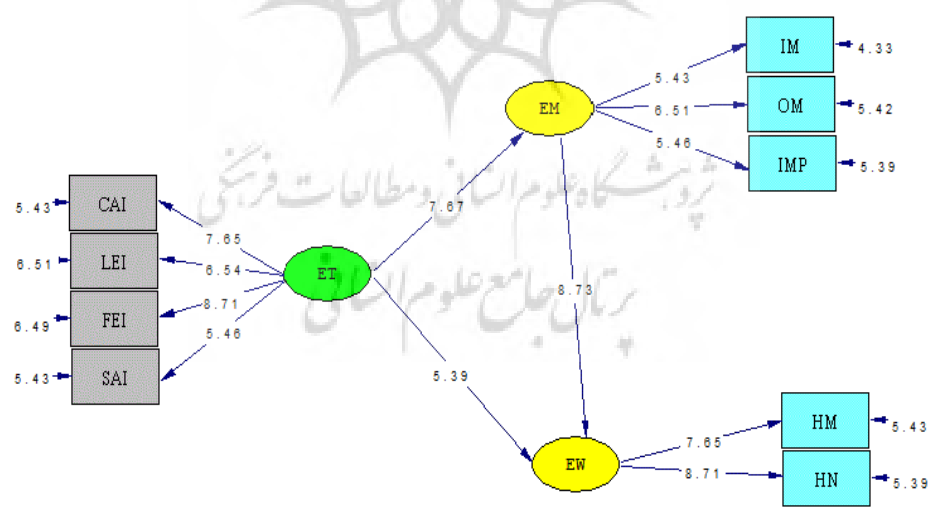
شکل ۵. آماره معناداری (t-value) نتایج تأیید مدل معادلات ساختاری فرضیات تحقیق
