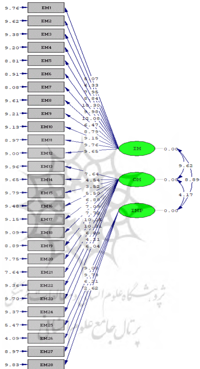
شکل ۲. آماره معناداری (t-value) تحلیل عاملی تأییدی پرسش نامه انگیزش تحصیلی
