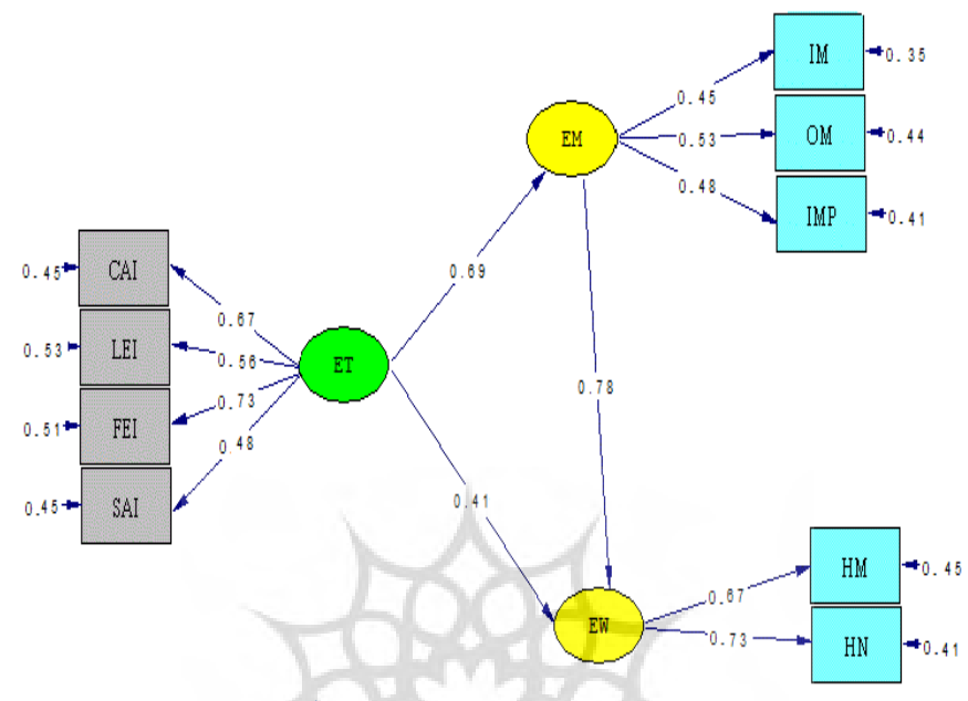
شکل ۴. نتایج تأیید مدل معادلات ساختاری فرضیات تحقیق
