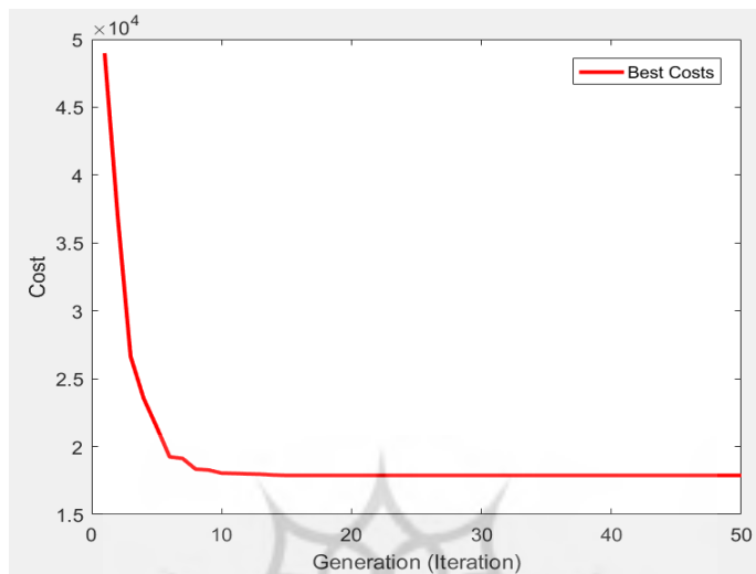
شکل ۱۱. نمودار همگرایی بدست آمده از بهینه سازی پرنده استوایی دریایی بهبود یافته برای اندازه مساله ۲۵ کار و ۱۵ ماشین
