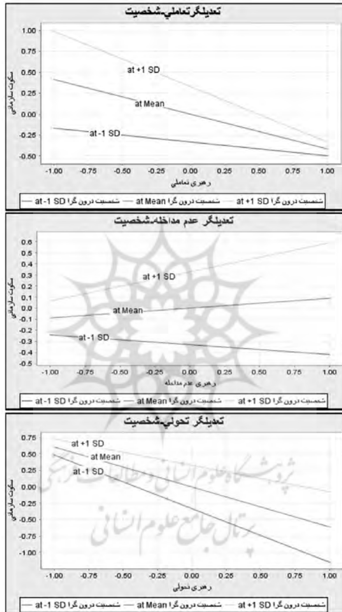
نمودار ۳. نتایج آزمون شیب ساده
