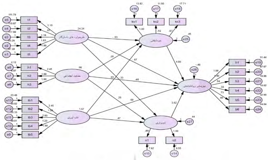
شکل ۲. مدل در حالت ضرایب استاندارد نشده
