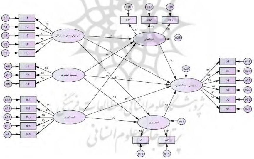
شکل ۳. مدل در حالت ضرایب استاندارد شده
